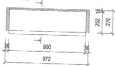
PUDORYS
