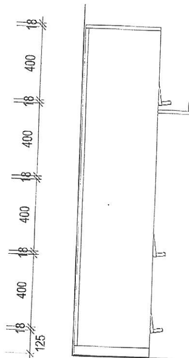
BOKORYSNÝ POHLED
