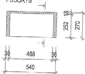
PŮDORYS
