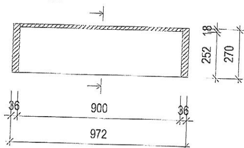
PŮDORYS
