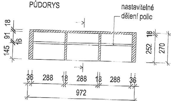
PUDORYS
