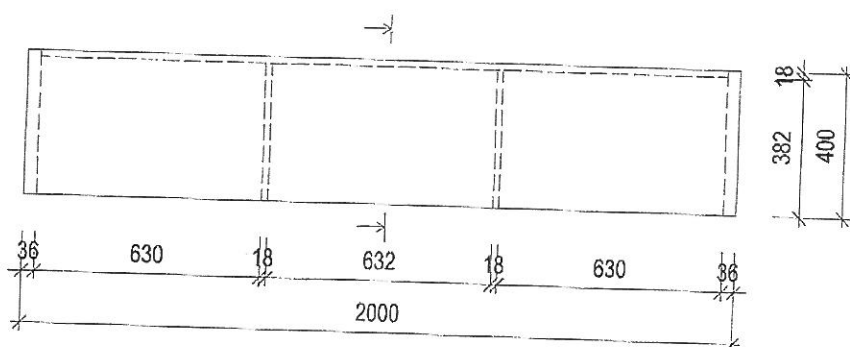
PŮDORYS
