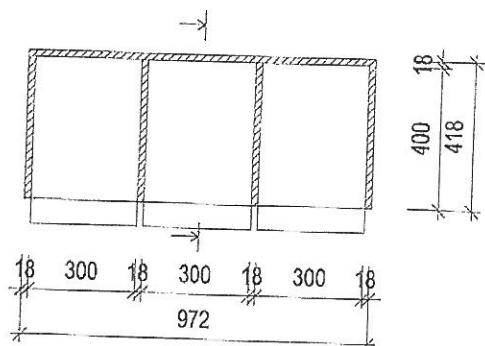
PŮDORYS
