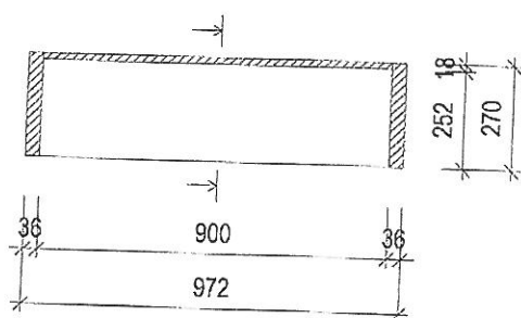
PŮDORYS
