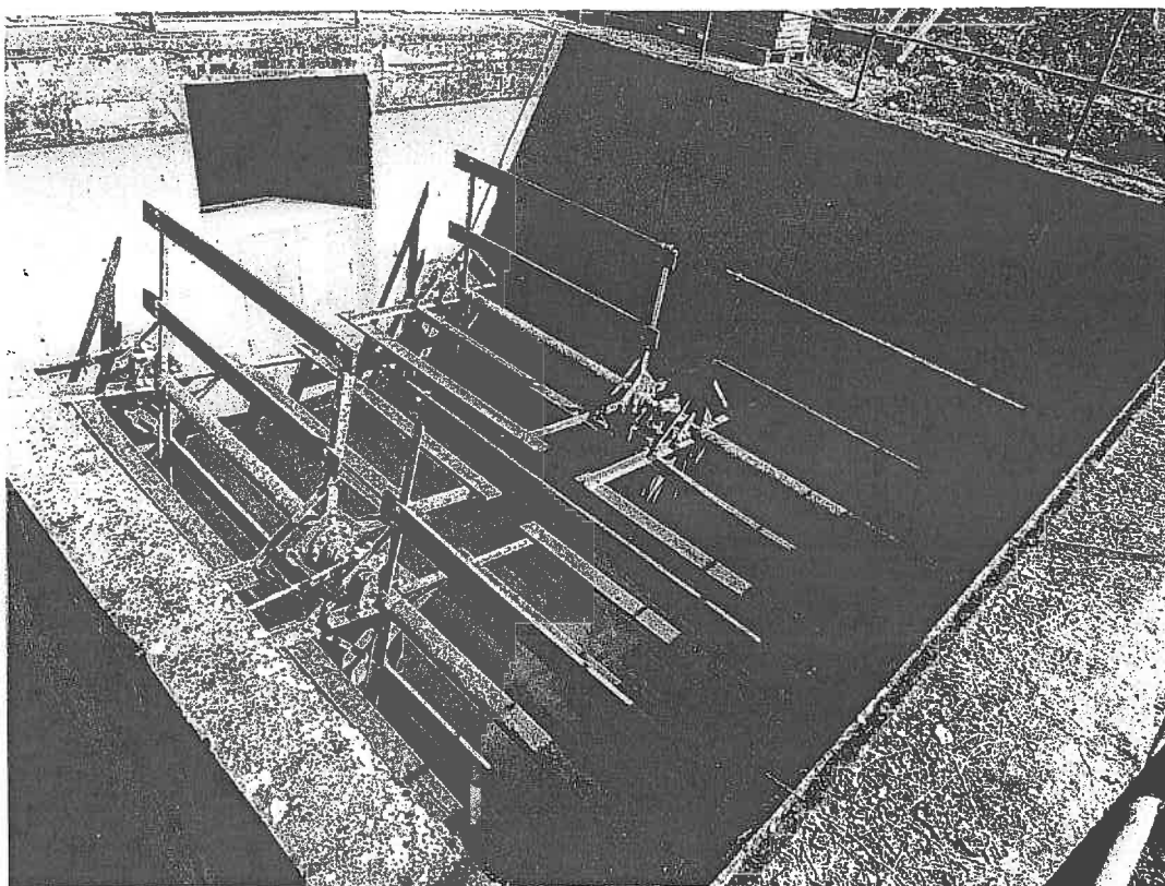
Stávající stav pomaluběžných míchadel v terciárním čištění.
