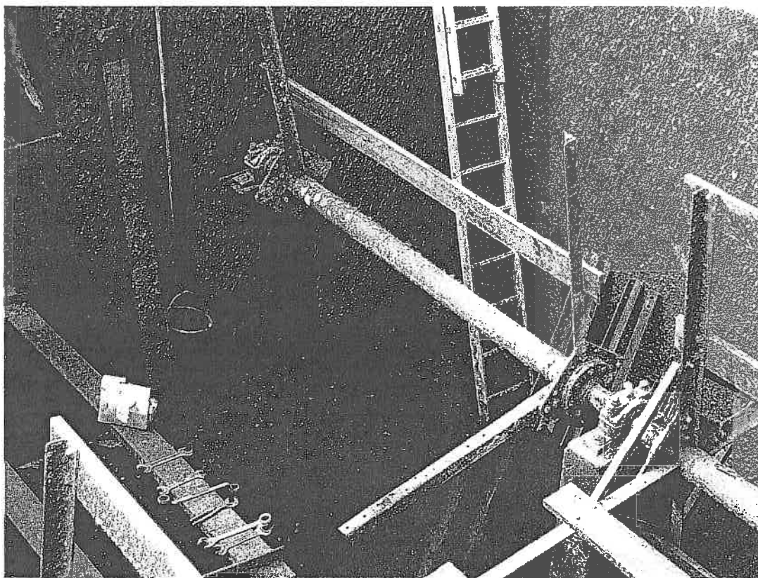
Pomaluběžná míchadla v terciárním čišťení – při poslední opravě.
